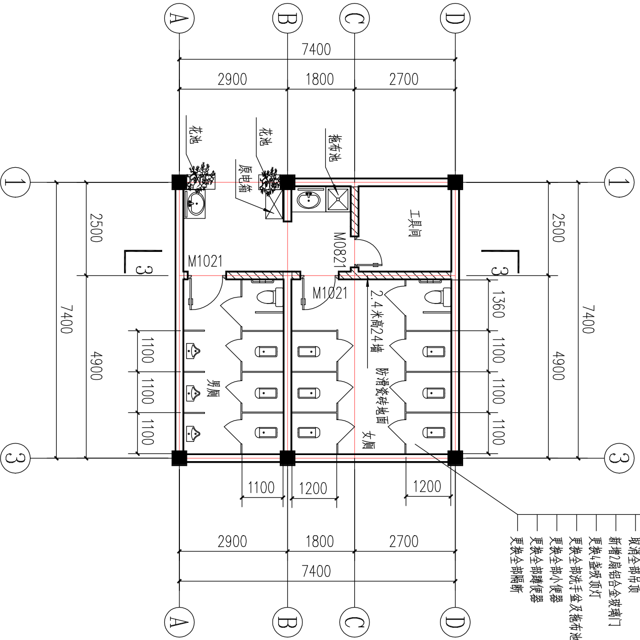
改造后公厕平面图
