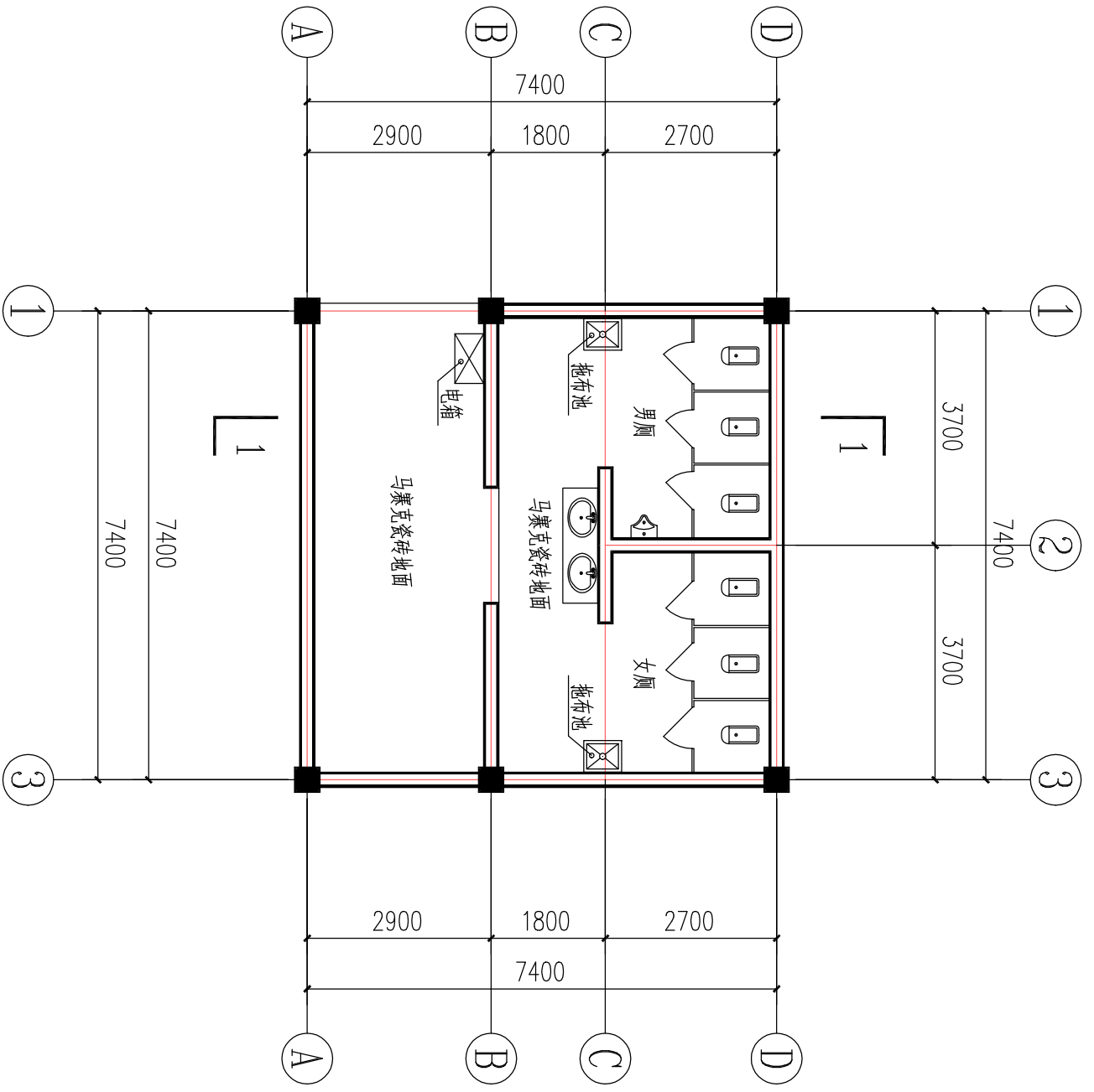
改造前公厕平面图
